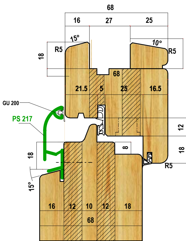
SEZIONE VERTICALE
