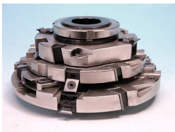
GRUPPI PER FINESTRE TOOLS FOR WINDOWS
