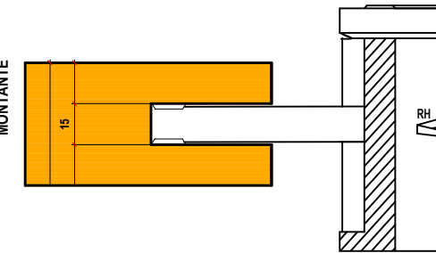
PS 06C INTERNO ANTA
