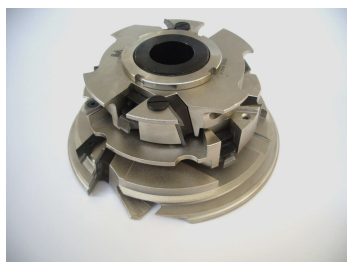
GRUPPI PER FINESTRE TOOLS FOR WINDOWS ARIA 4 - 12
