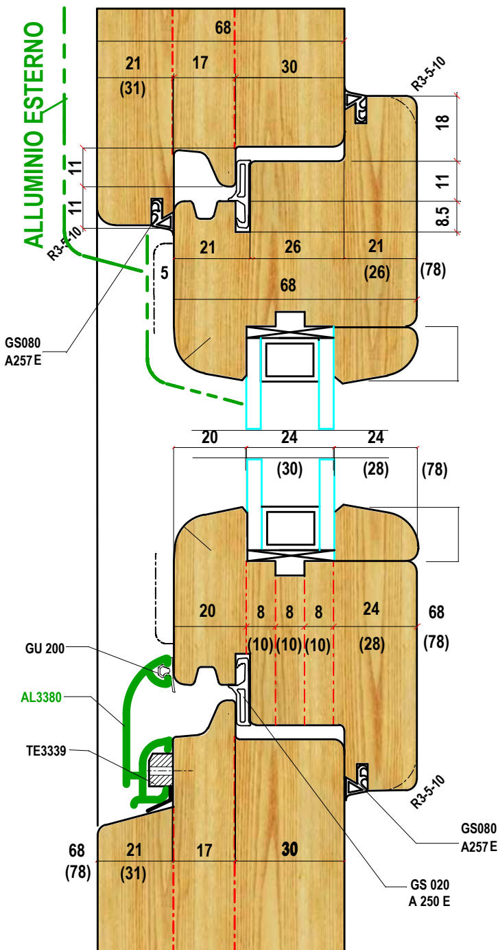
SEZIONE VERTICALE
