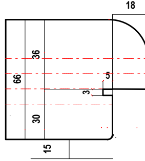
06 PROFILO INTERNO ANTA
