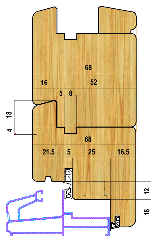
PORTA FINESTRA
