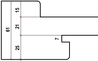
03 TENONE TELAIO
