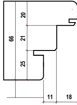
09 SQUADRATURA ANTA
