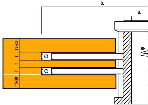
PS 02 TENONE MONTANTI ANTA
