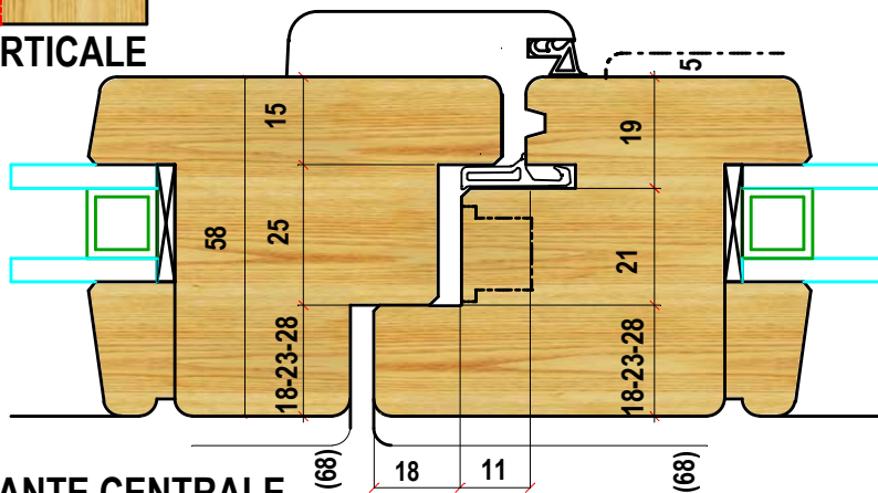
MONTANTE CENTRALE
