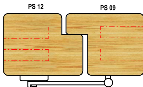
CHIUSURA CENTRALE
