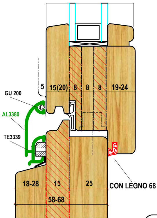
SEZIONE VERTICALE
